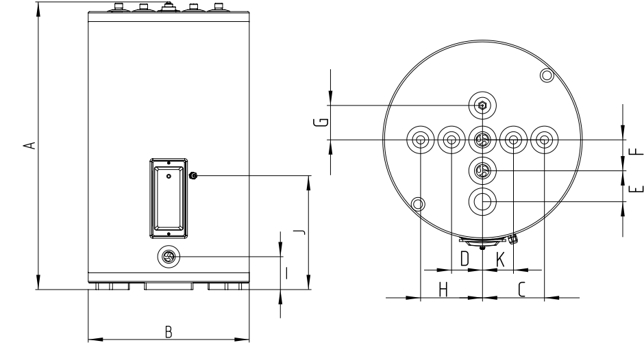
Рис.4 Габаритные размеры водонагревателя ZOTA E-HOT 150 Up
