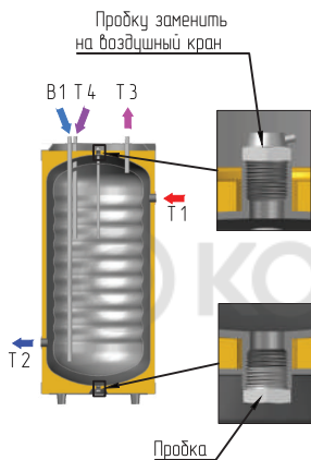
Рис. 5 Напольный монтаж
