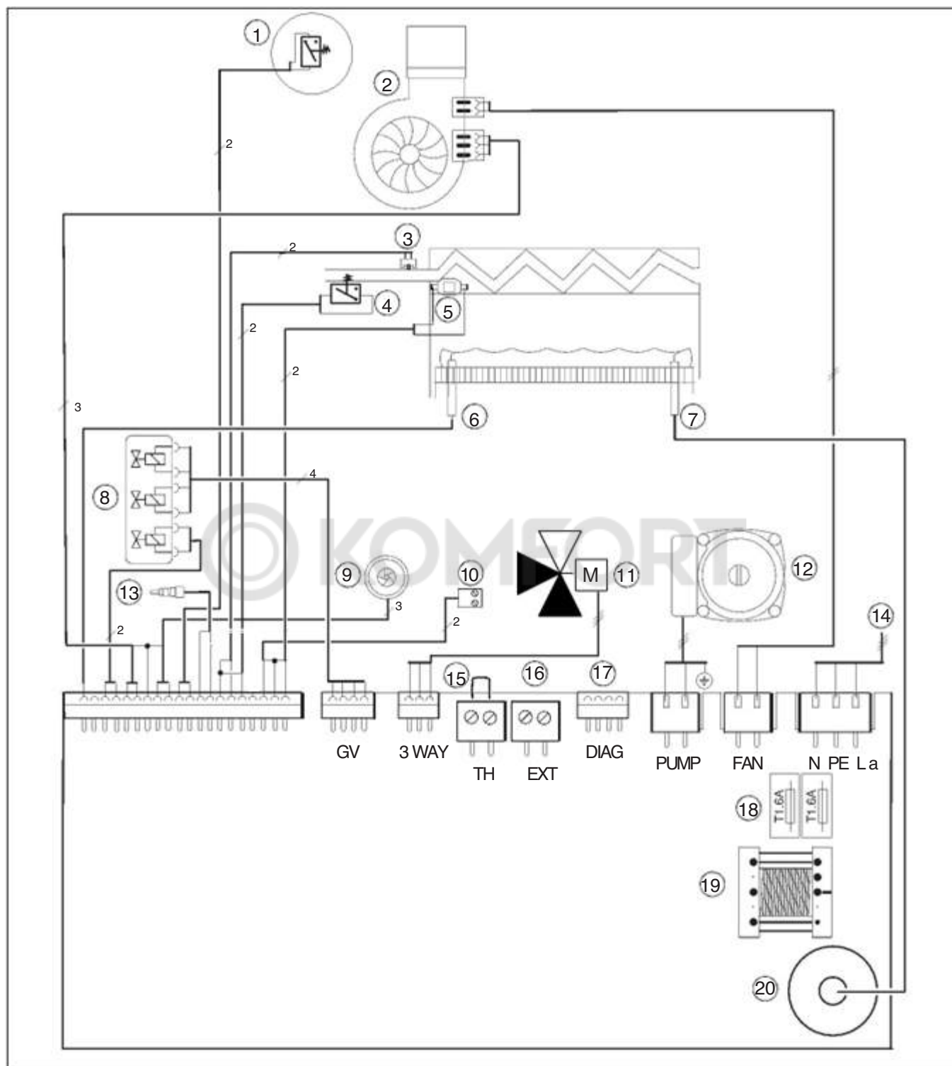
Рис. 41 Электрическая схема
