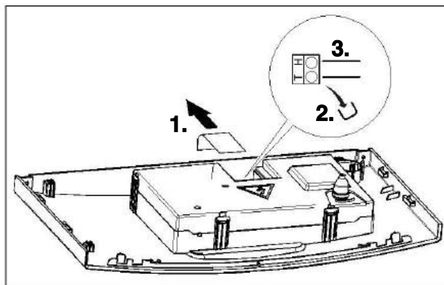
Рис. 21 Подключение регулятора
