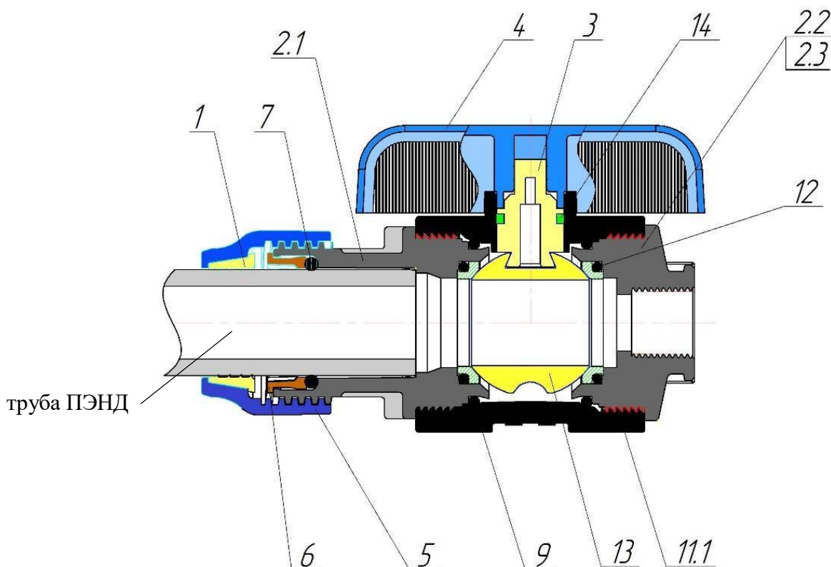
Рисунок 1. Конструкция крана шарового с Ø20 по Ø32
