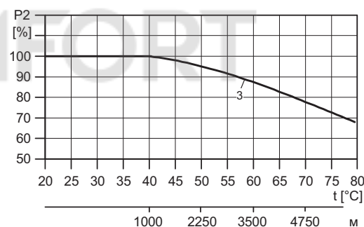
Рис. 33. Зависимость между мощностью на валу электродвигателей MGE (P2) и температурой окружающей среды.
