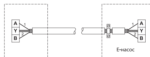
Рис. 41 Соединение экранированным 2-жильным кабелем
