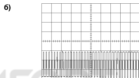
Рис. 45 а) ток электродвигателя и напряжение б) участок напряжения электродвигателя
