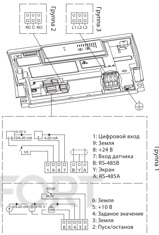
Рис. 37 Схема подключения
