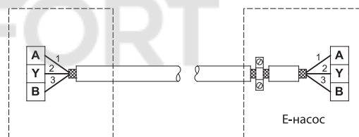
Рис. 40 Соединение экранированным 3-жильным кабелем – металлическая скоба только на конце Е-насоса
