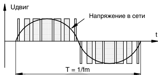
Рис. 44 Напряжение, подаваемое на электродвигатель
