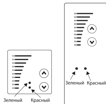
Рис. 24 Панели управления Е-насоса
