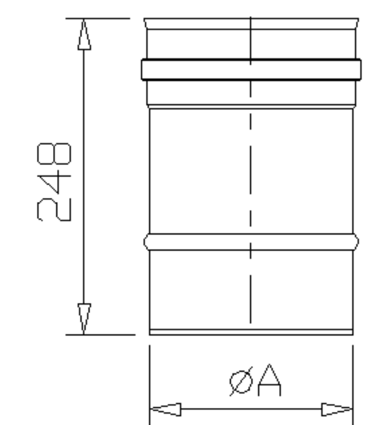
fu 04 Труба 250 мм
