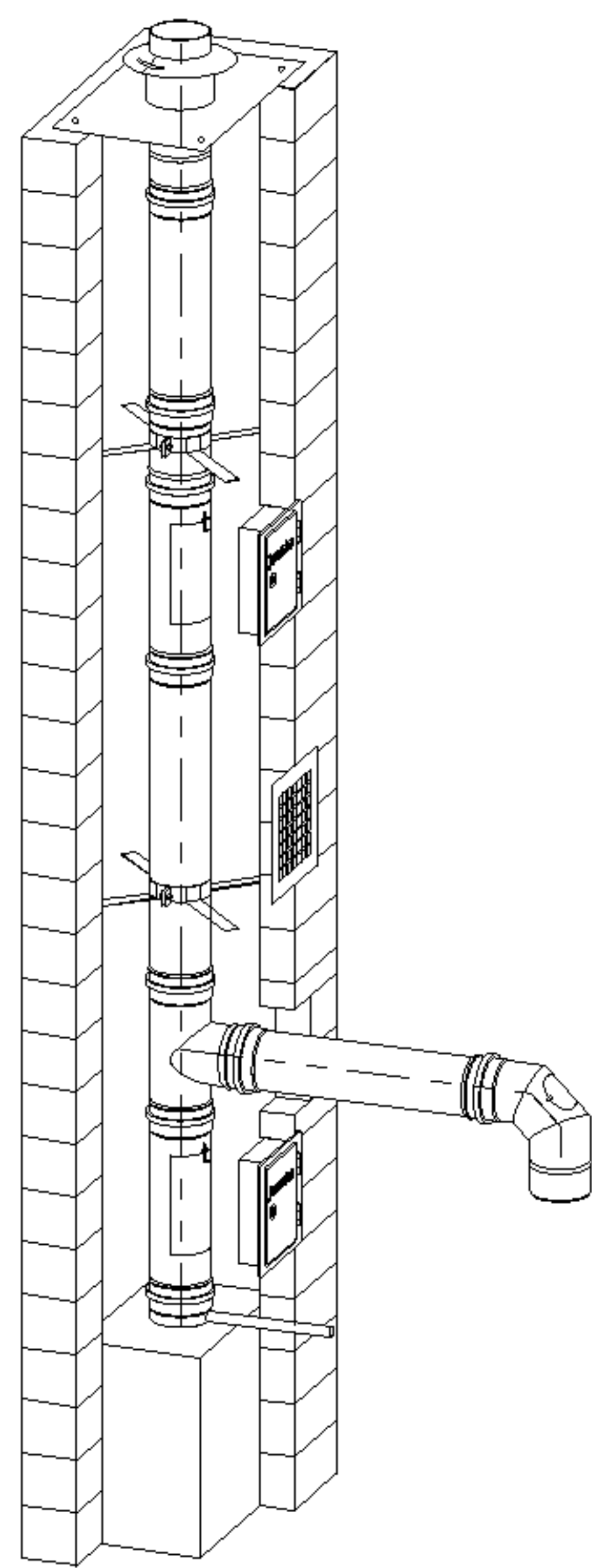
Рис. 3: стандартное устройство
