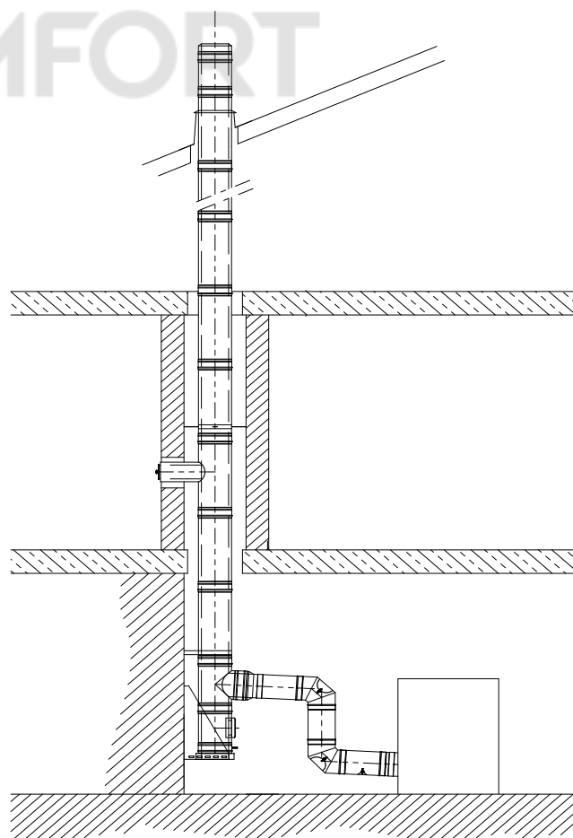
Рис. 13b: внутренняя установка
