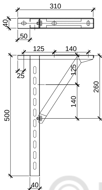
DW 392 Стеновая консоль тип II, длина 500 мм
