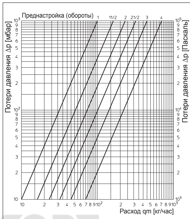
Диаграмма 11 „Duo“- рисоединительная насадка для двухтрубных систем (межосевое расстояние 35 мм) и термостатический вентиль серии „А“, DN 15.
