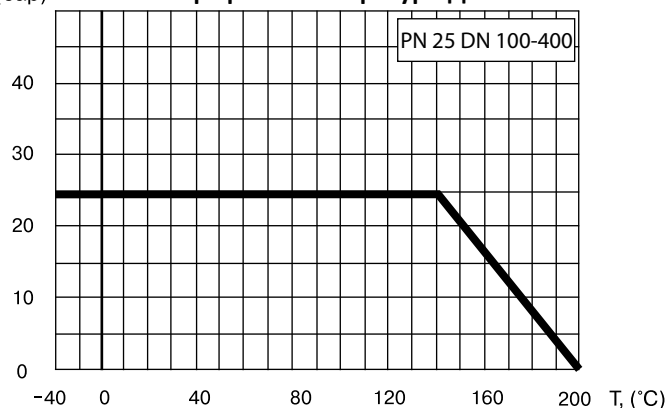
График «Температура-Давление»
