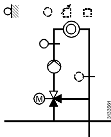
Смесительный контур
