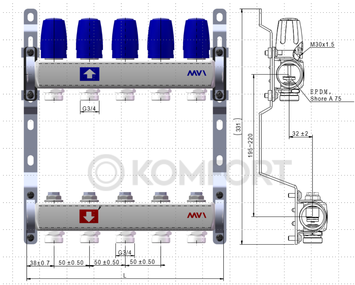
Коллекторный блок из нержавеющей стали без расходомеров
