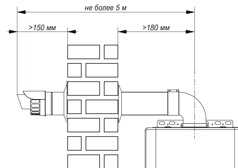
Рисунок 9. Коаксиальный дымоход.
