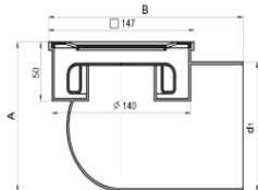
а) с сухим затвором
