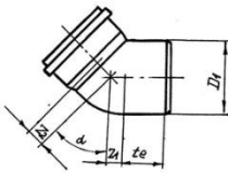
Рисунок 7. Отвод
