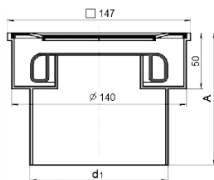
Рисунок 12. Трапы с вертикальным выпуском
