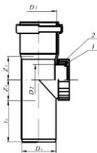
Рисунок 9. Ревизия (1-уплотнение; 2-крышка ревизии)
