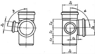
Рис 5.1. Крестовина двухплоскостная
