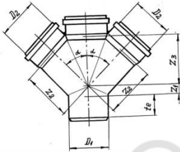
Рис 4. Крестовина одноплоскостная
