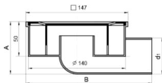
б) с гидрозатвором
