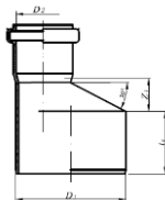
Рисунок 10. Переход редукционный
