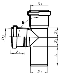
Рисунок 13. Тройники
