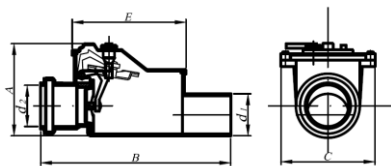
Рисунок 14. Обратные клапана
