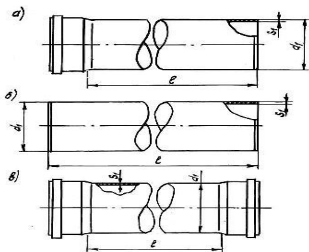
Рисунок 1 - Трубы.
