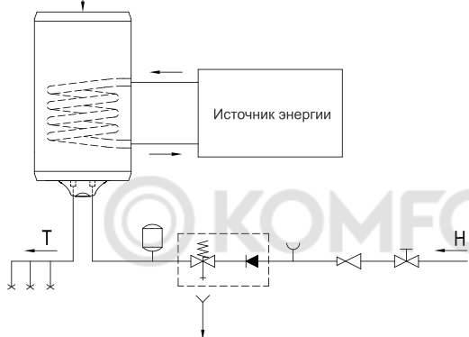
Закрытая (накопительная) система
