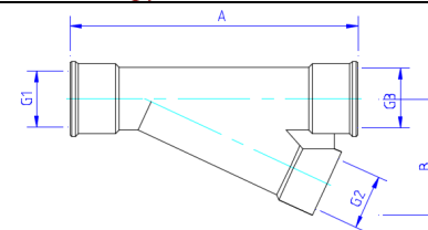
VTr.136 Тройник косой 25° для погружной гильзы В-В-В
