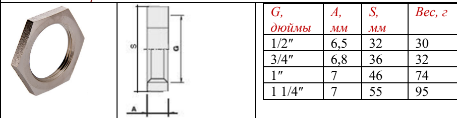
VTr. 656 Контргайка по ГОСТ В
