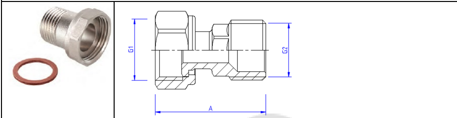
VTr. 613 Соединитель с накидной гайкой В-Н
