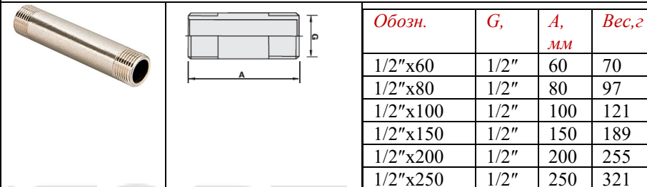
VTr. 653 Сгон Н-Н
