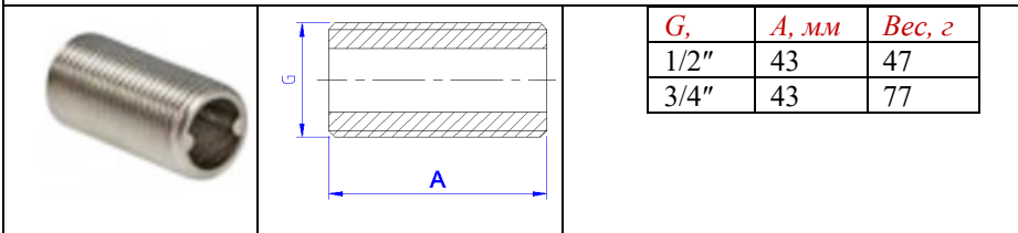
VTr. 651 Ниппель под сгонный ключ Н
