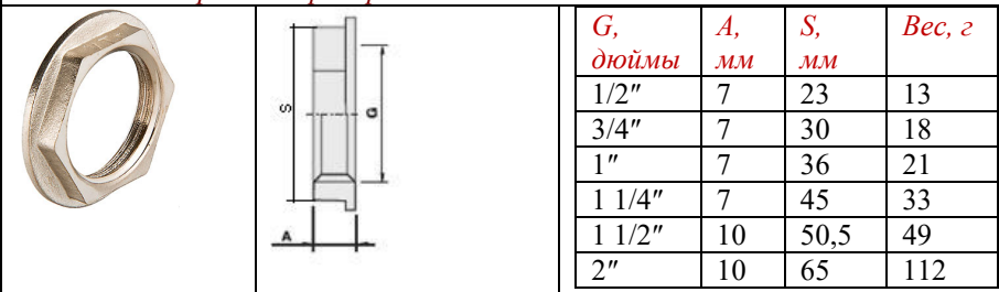
VTr. 656 Контргайка по ГОСТ В
