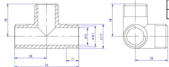
VTr. 661 Крестовина двухплоскостная Н-Н-Н
