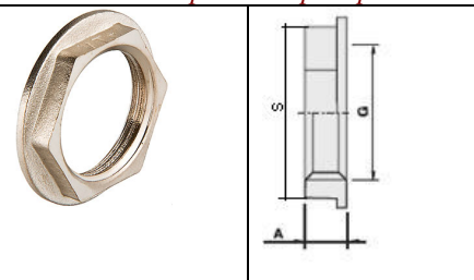
VTr. 656 Контргайка по ГОСТ В
