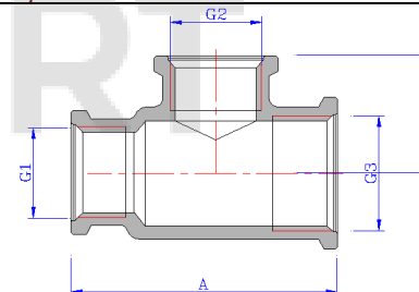
VTr. 750.RN Тройник переходной В-В-В
