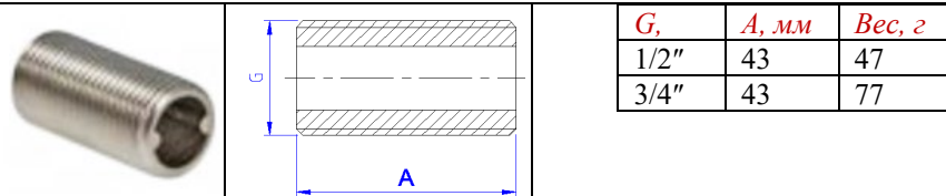
VTr. 651 Ниппель под сгонный ключ Н
