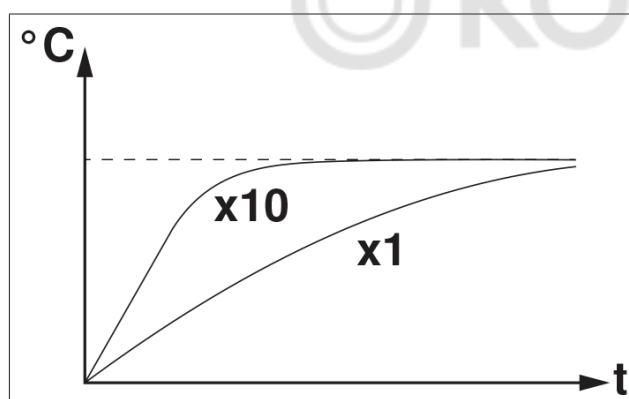
Рис. 13: Температурный режим
