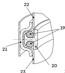
Разрез по месту соединения полукорпусов
