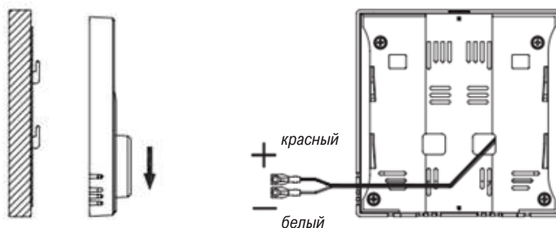
Рисунок 15. Подключение пульта управления NCTR-60R.
