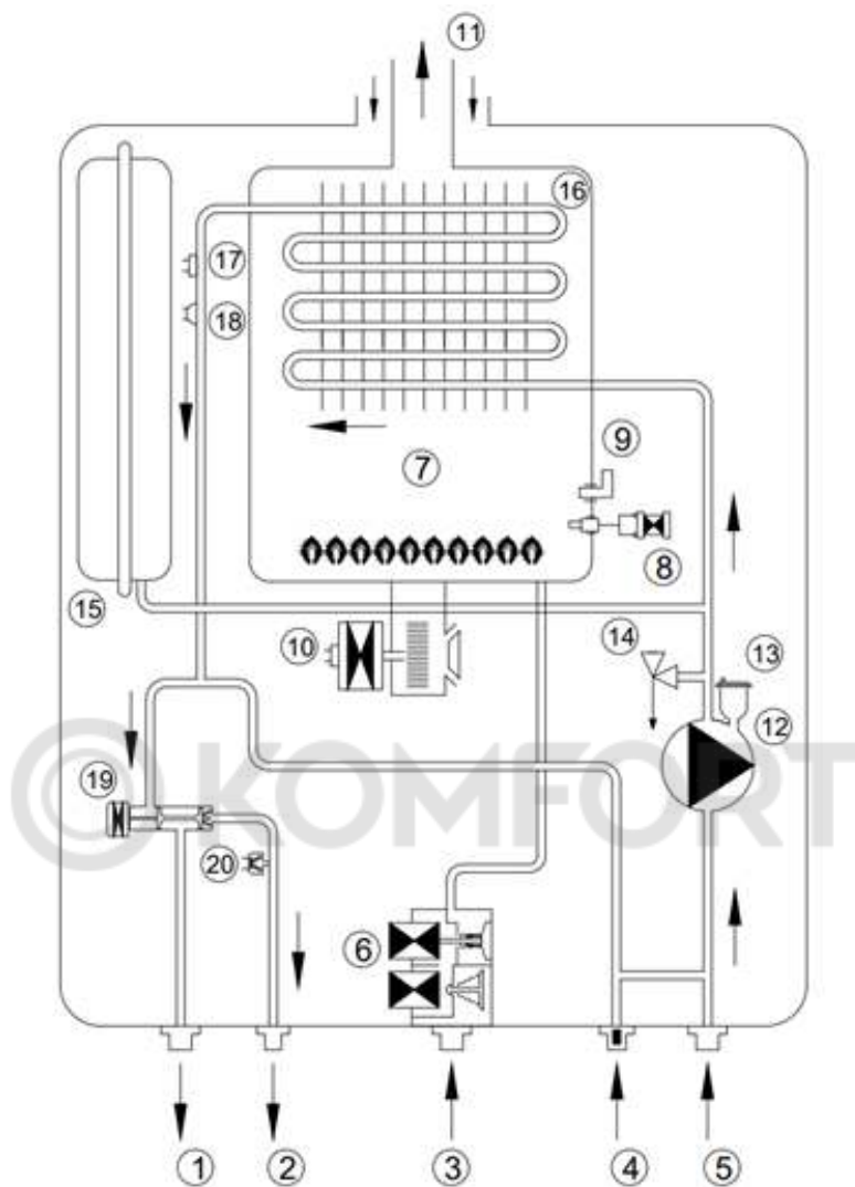
Рисунок 3. Функциональная схема котла.
