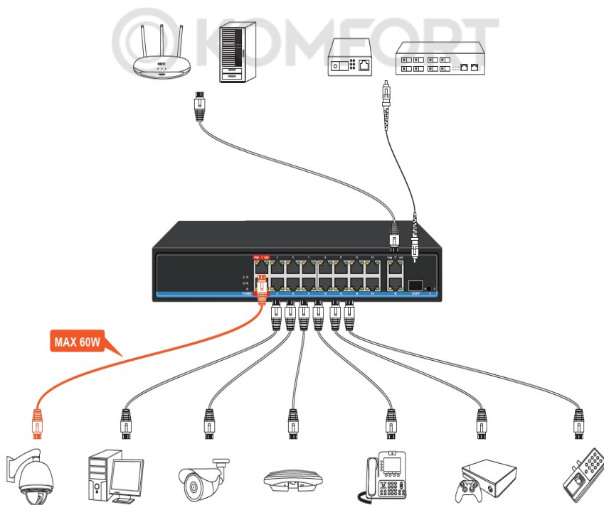
Рисунок 6 – Схема подключения устройств к коммутатору
