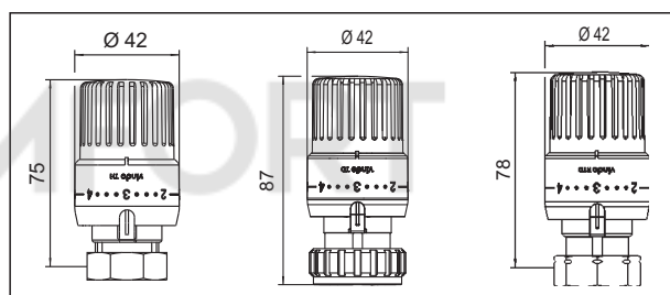
Термостат „vindo TH“
