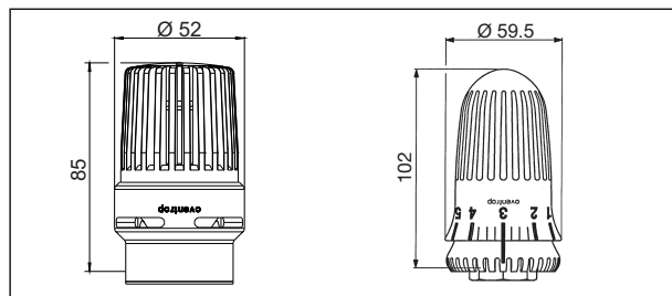
Термостат „Uni LHB“
