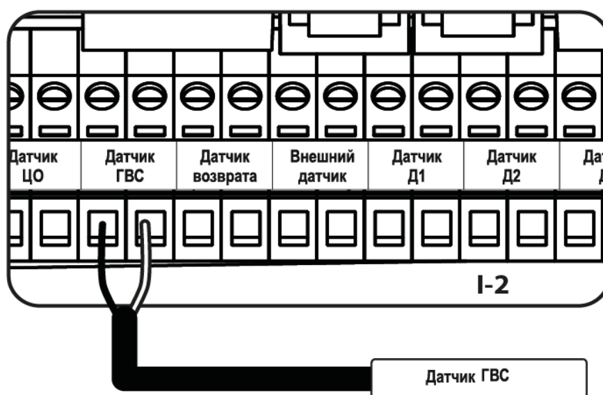
Подключение датчика ГВС
