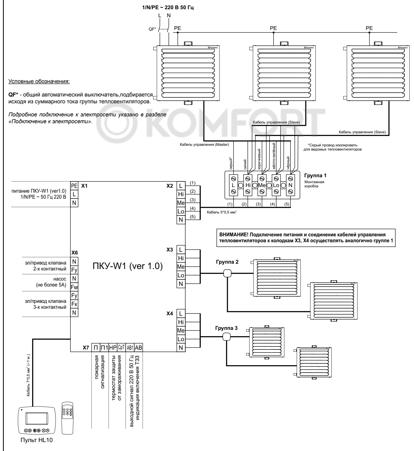
Схема подключения групп тепловентиляторов к ПКУ-W1 (ver1.0)
