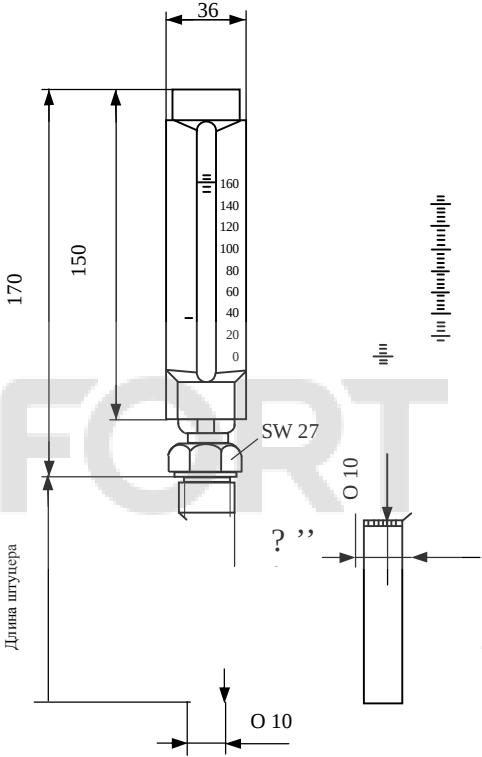
Термометр MTG
