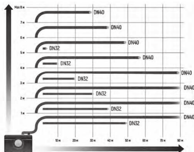
Рис. 20 Максимальная длина напорного трубопровода
