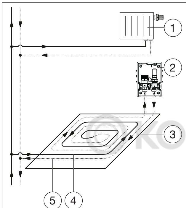
Рис. 6: Подключение
