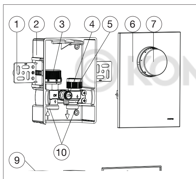
Рис. 2: Конструкция „Unibox E RTL“
