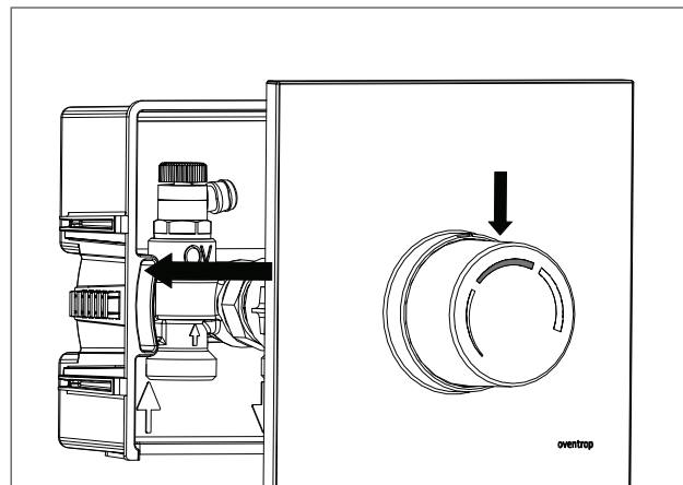
Рис. 9: Надеть крышку
