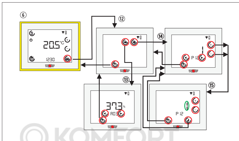
Рис. 10.5 Меню
