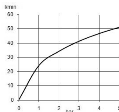
График расхода воды
