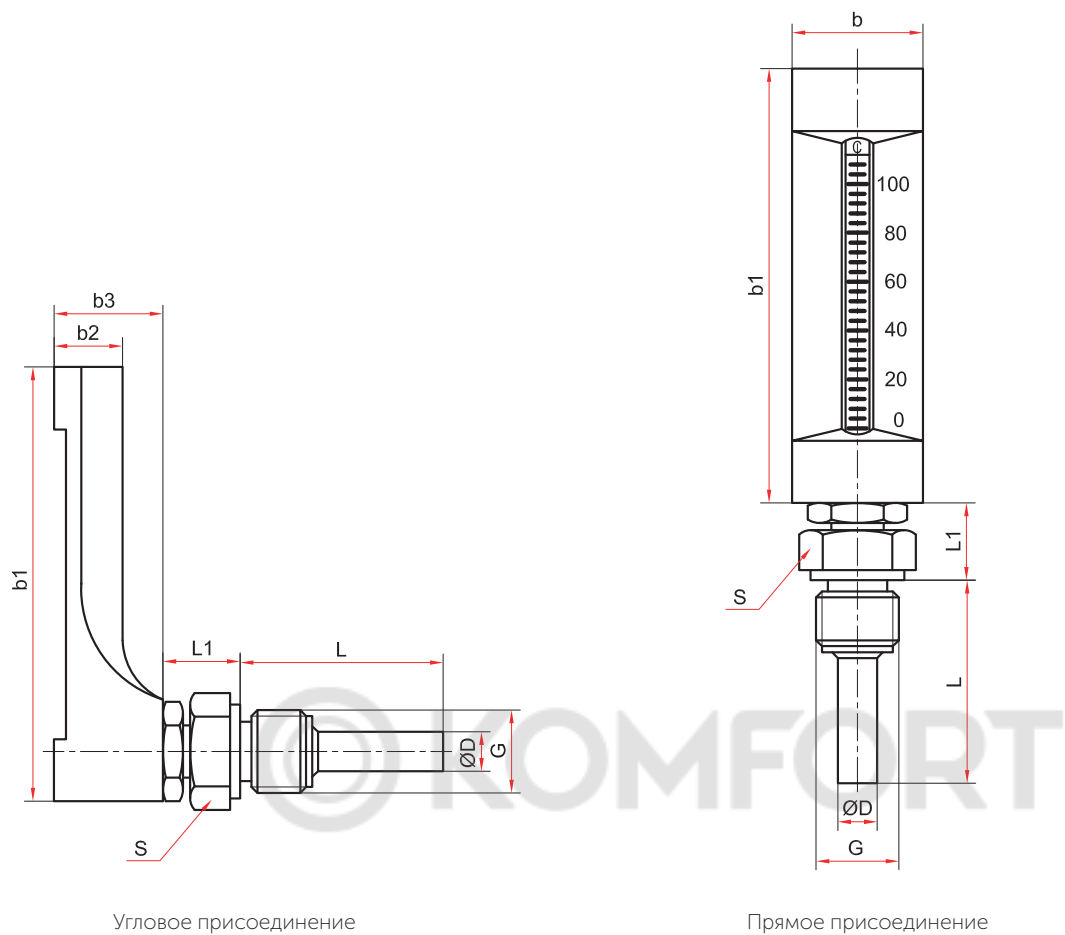
Основные размеры (мм), вес (кг)
