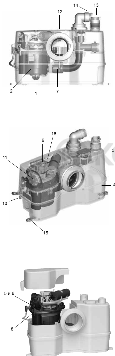
Sololift2 WC-1
