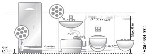
Рис. 23 Пример монтажа
