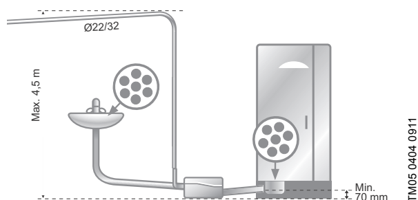
Рис. 41 Пример монтажа
