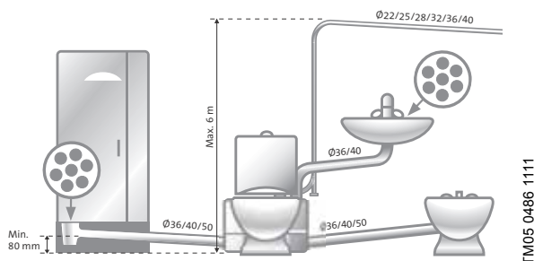
Рис. 14 Пример монтажа
