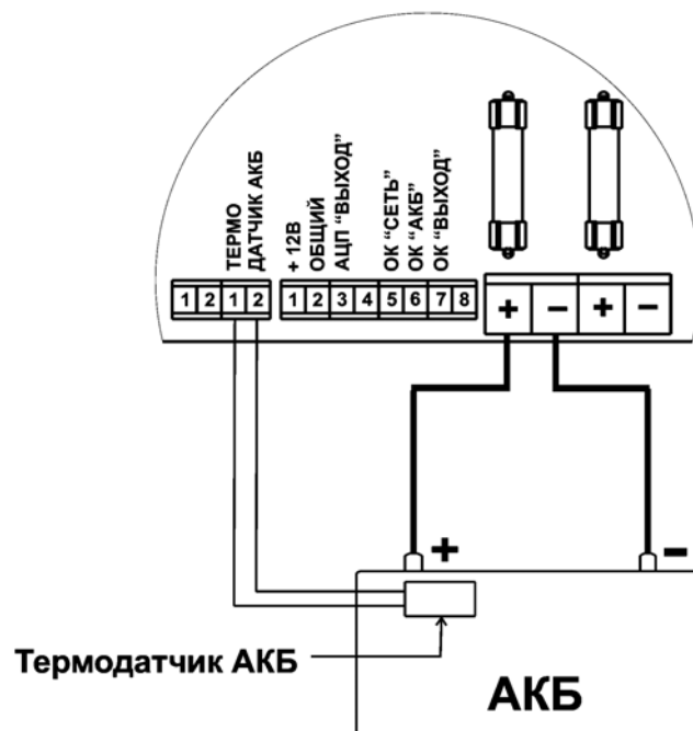
Рисунок 5. Подключение АКБ и термодатчика.
