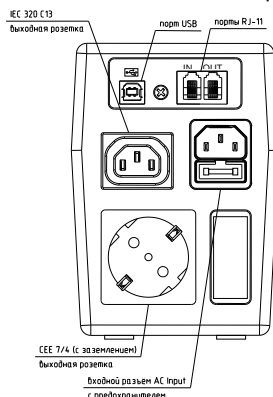
Рисунок 1 - Задняя панель ИБП
