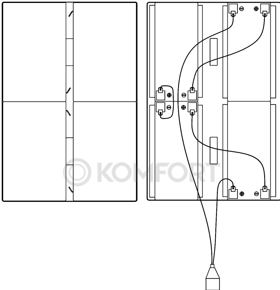
Рисунок 6 — размещение АКБ в лотке
