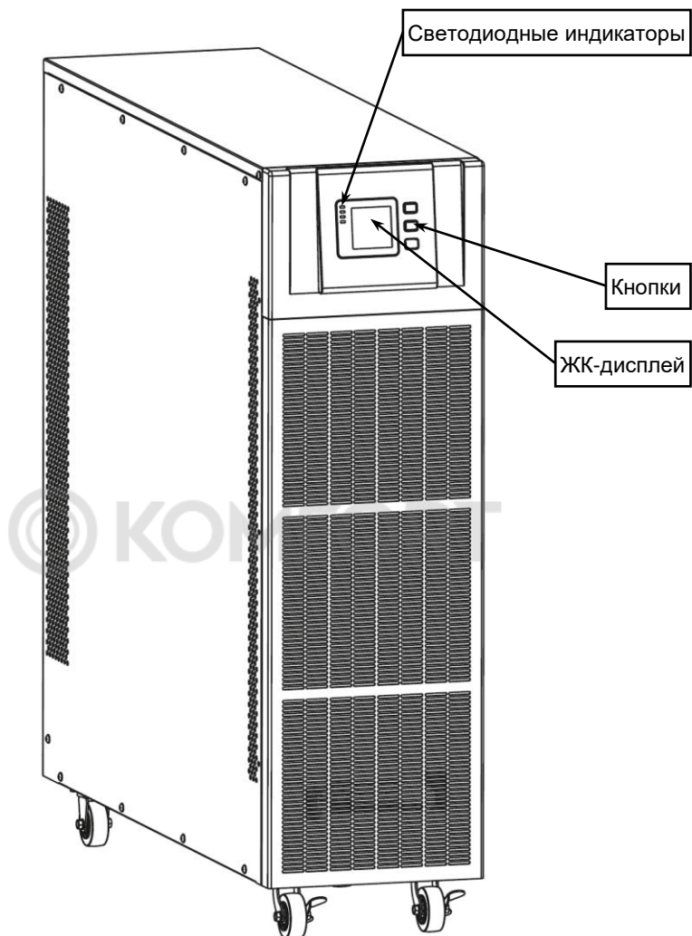
Рисунок 1 - Общий вид изделия спереди и слева
