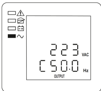
Рисунок 13 — ЖК-дисплей: фаза С, выходное напряжение и частота
