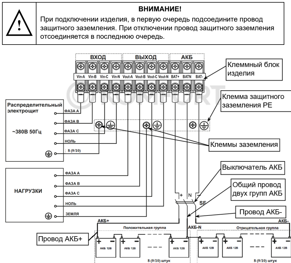
Рисунок 23 — Схема подключения изделия и монтажа аккумуляторной батареи.
