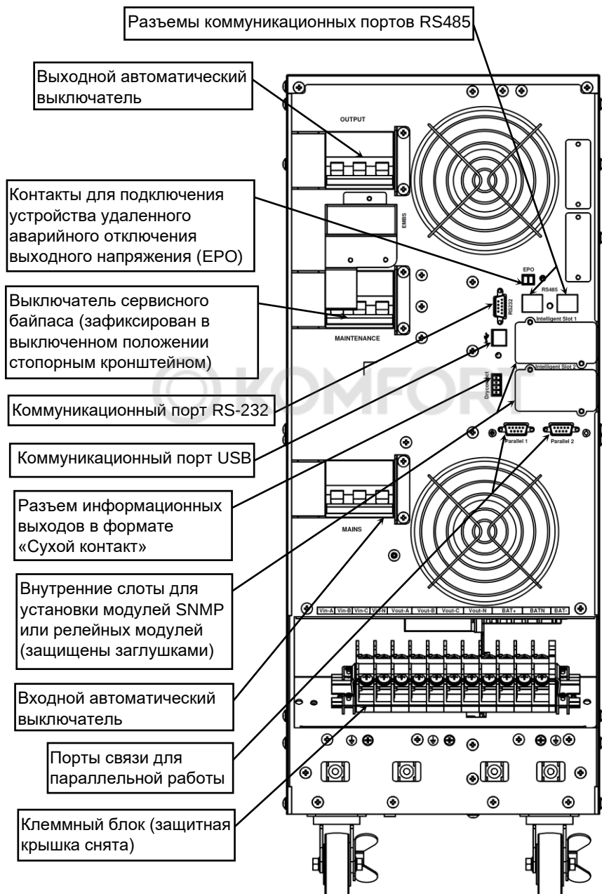
Рисунок 2 — Общий вид задней панели изделия со снятой крышкой клеммного блока
