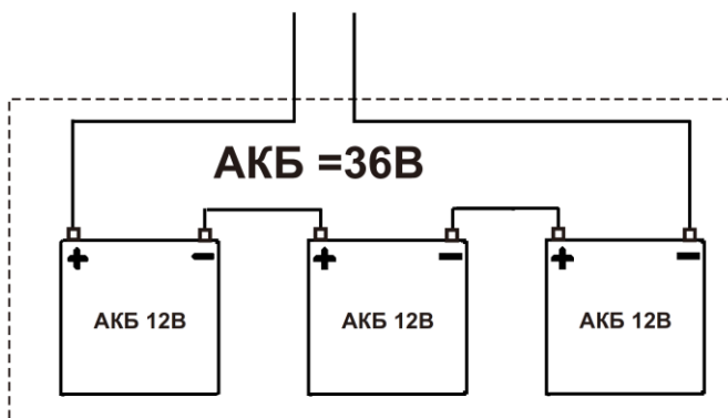
Рисунок 6 — Схема монтажа аккумуляторной батареи.
