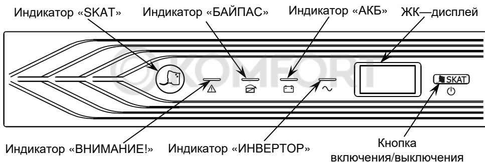
Рисунок 7 — Общий вид передней панели изделия
