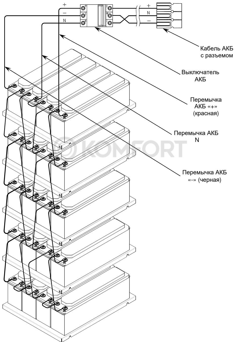
Рисунок 4 — Пример монтажа и размещения АКБ на полках комплекса.
