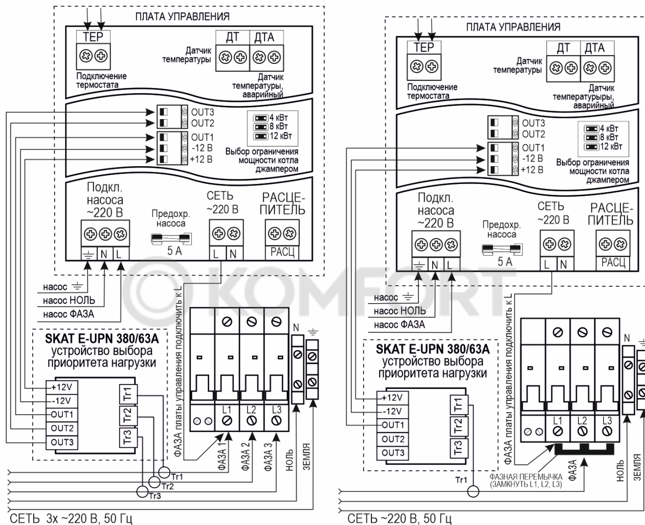
Схема подключения электрокотла к сетям ~220 В и 3х~220 В
