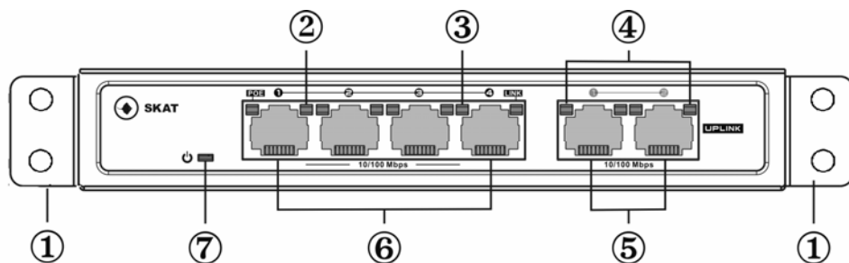
Рисунок 4 – передняя панель коммутатора
