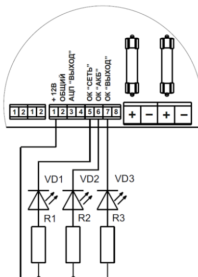
Рисунок 5 – Подключение внешних индикаторов
