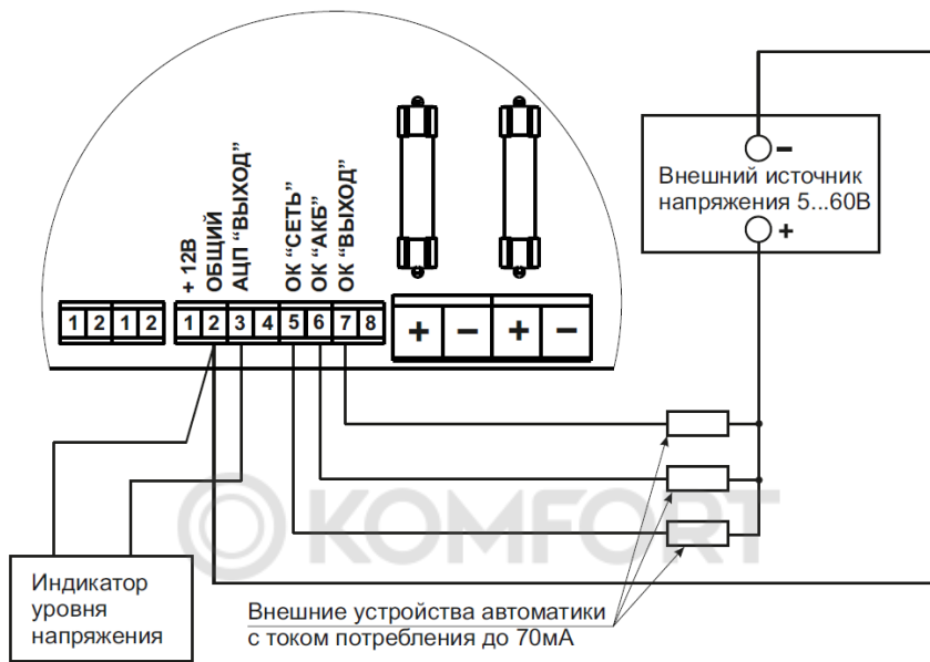
Рисунок 4 – Подключение внешних устройств автоматики.
