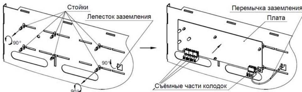
Рисунок 3 - Установка платы
