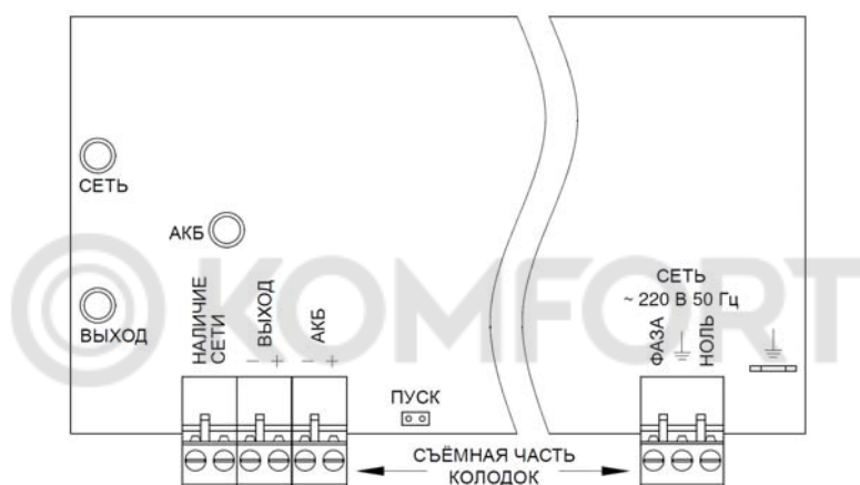
Рисунок 2 - Общий вид платы
