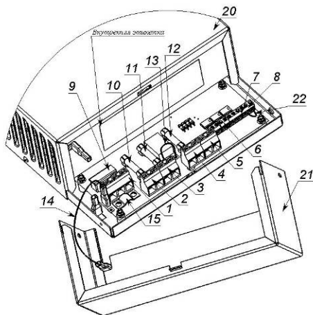
Рисунок 1- вид изделия со снятым кожухом монтажного отсека
