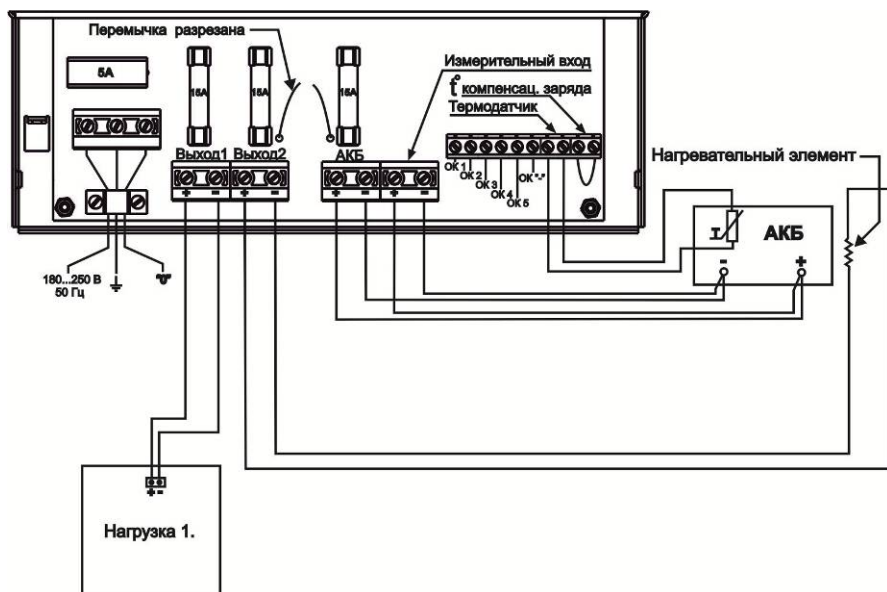
Рисунок 5 – подключение нагревательного элемента
