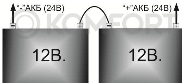
Рисунок 8 – схема последовательного соединения двух аккумуляторов
