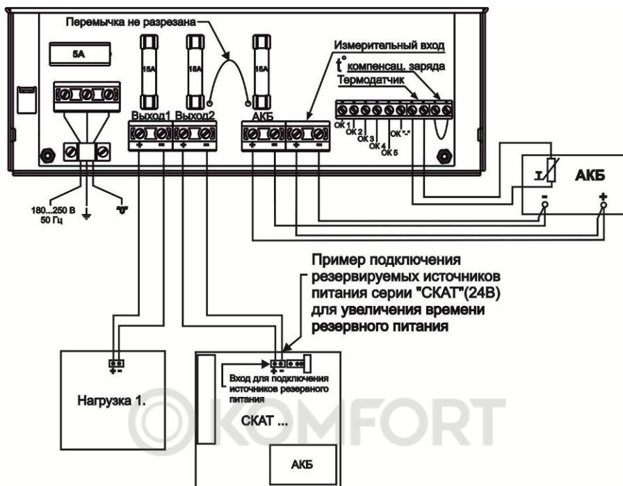
Рисунок 4 – подключение изделия
