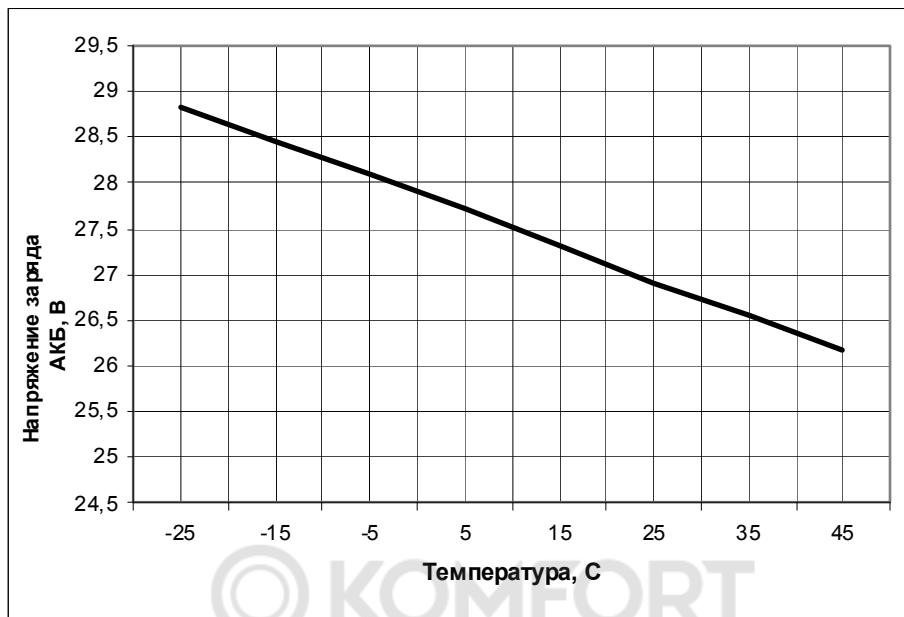
Рисунок 3 – зависимость напряжения заряда АКБ от температуры
