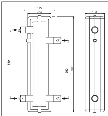
Гидрострелка Ду32
