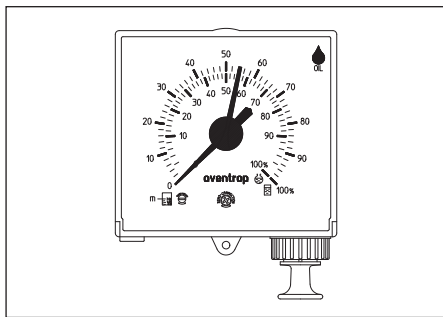
Пневматический указатель уровня
