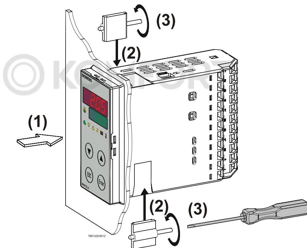
Иллюстрация 3: Установка в вырез панели управления
