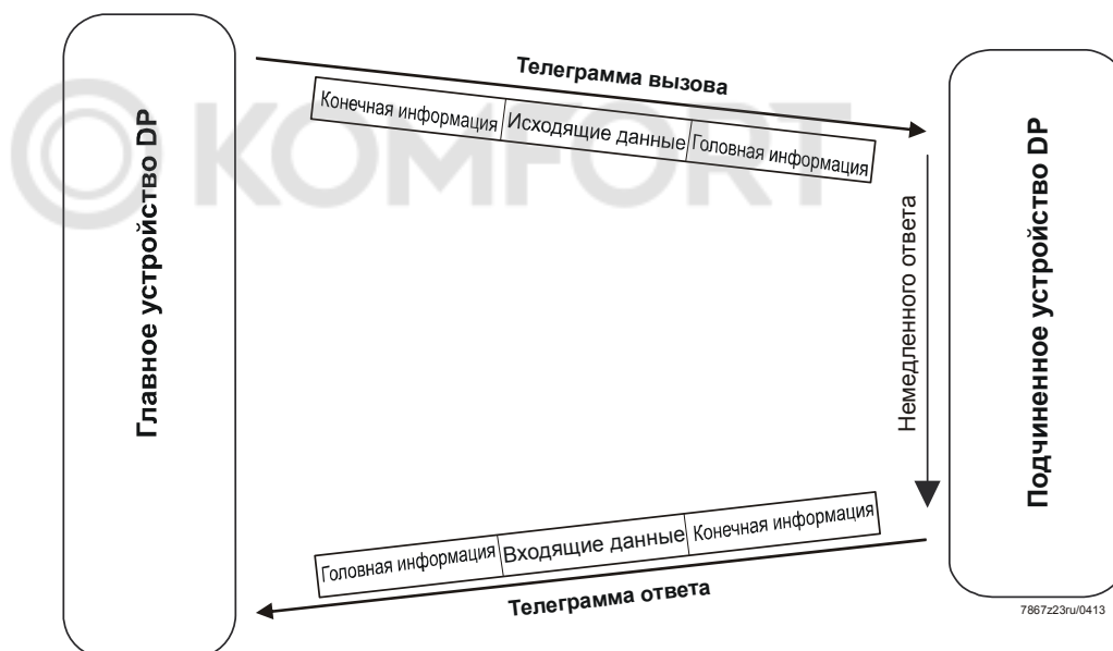
Иллюстрация 40: Передача полезных данных по шине Profibus-DP
