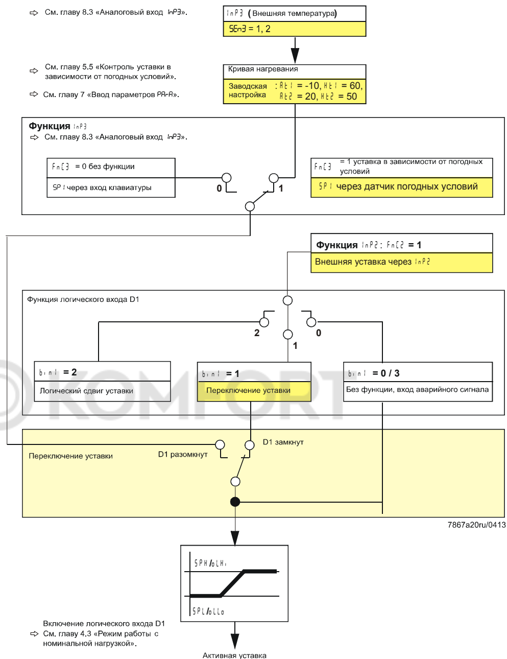
График 13: Переключение уставки SP1 /внешняя уставка
