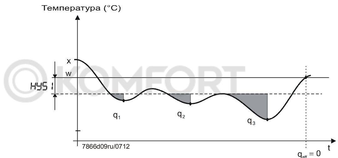
Иллюстрация 17: Программируемый цикл горелки, порог срабатывания (q)
