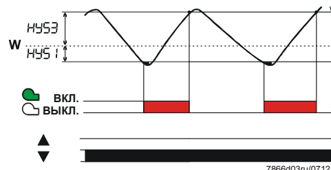
Иллюстрация 6: Программируемый цикл контроллера системы отопления
