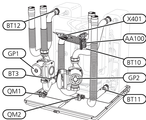
Компрессорный модуль EP15
