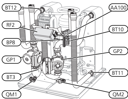
Компрессорный модуль EP14
