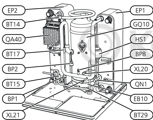
Компрессорный модуль EP15
