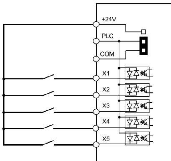
Управление входами по схеме PNP
