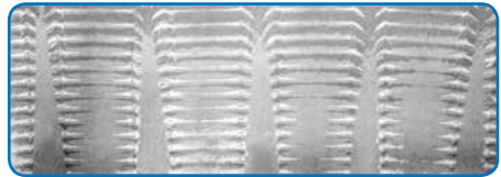
Расширение без поворота головки (неправильно)
