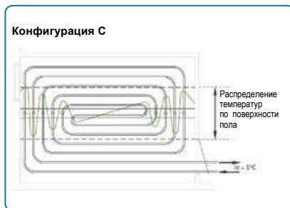
Вариант укладки – Спираль. Распределение температуры по поверхности пола
