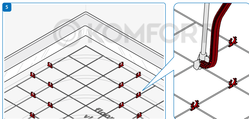
При использовании клипс закрепите их на армирующей сетке
