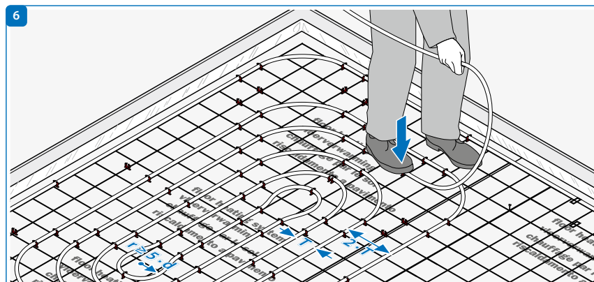
Разложите трубу с необходимым шагом и закрепите ее
