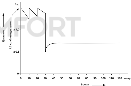
Порядок проведения гидравлических испытаний водой
